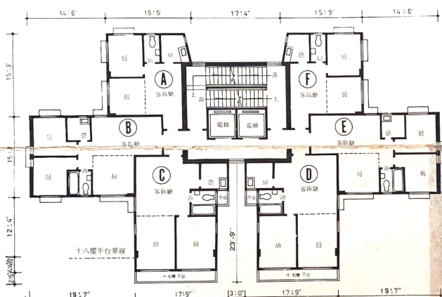
十七樓至十八樓平面圖
