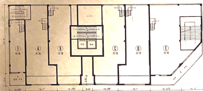
閣樓平面圖
