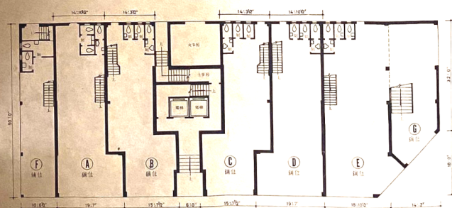
地下平面圖
