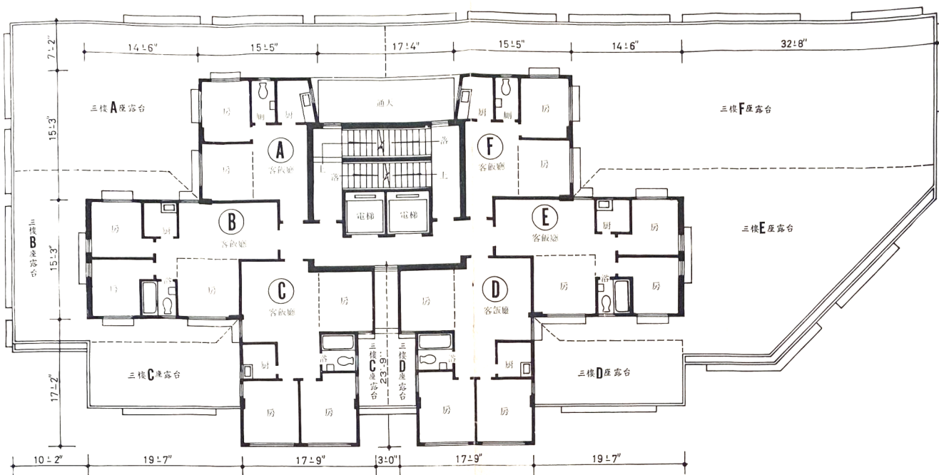
三樓至十六樓平面圖
